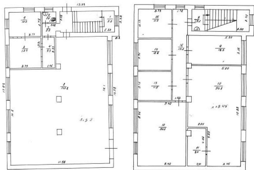
План приміщення
